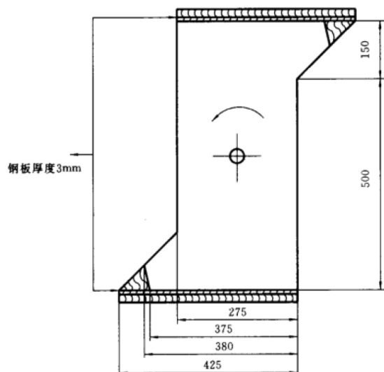
图 1 滚筒
