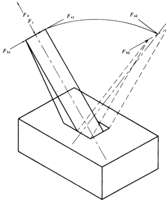
图 3 加力方法
