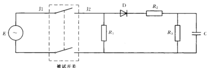
图4 试验电路
