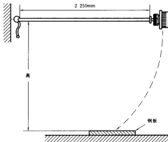
图 2 撞击试验
