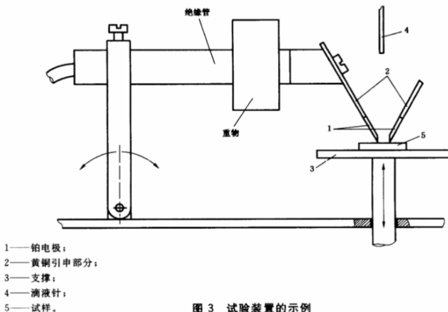
图 3 试验装置的示例
