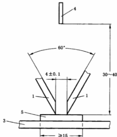
图 2 电极装置
