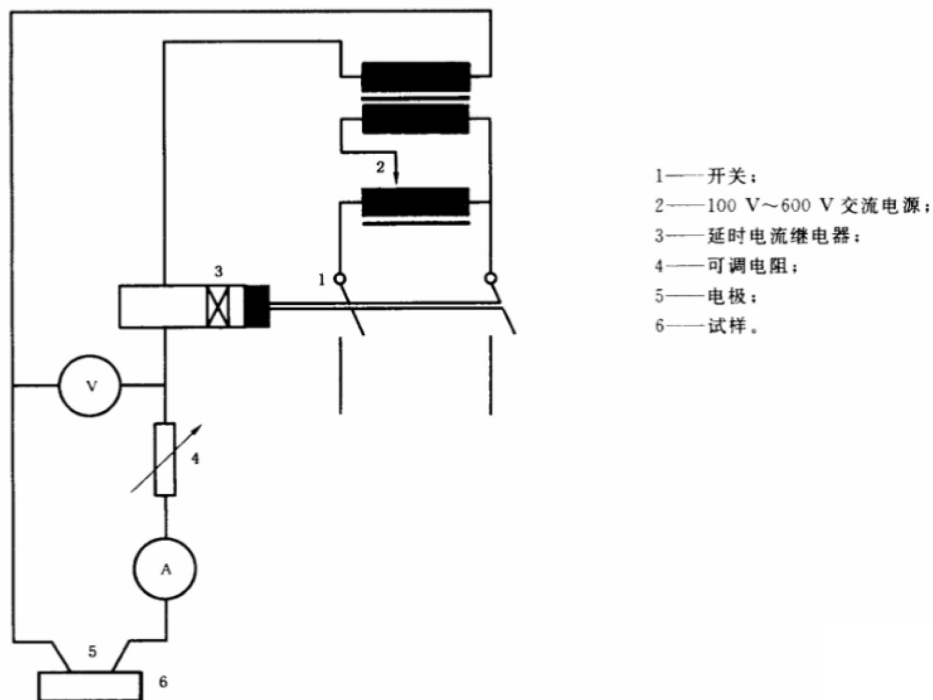
图 4 试验电路的示例
