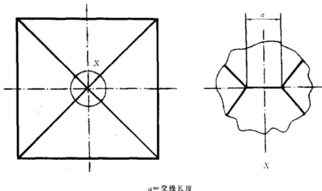
图 2 压头锥顶交线的示意图
