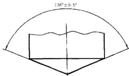
图 1 金刚石棱锥体的锥角
