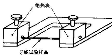
图 D. 1 焊球可焊性试验装置
